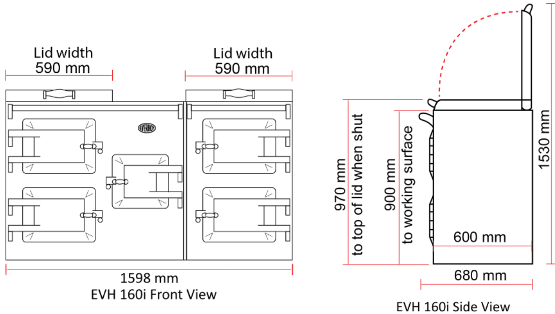
EVH160i dimensions
